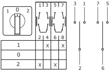
TIPO THS-U2 - 2 PÓLOS
