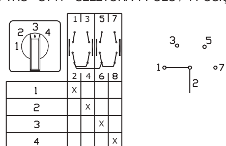
TIPO THS - ST41 - SELETORA 1 PÓLO / 4 POSIÇÕES
