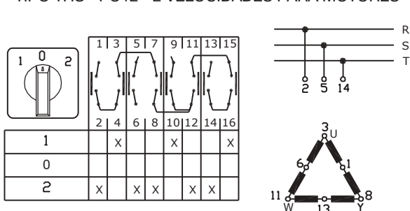
TIPO THS - PO12 - 2 VELOCIDADES PARA MOTORES
